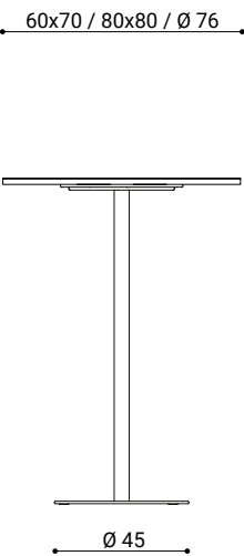
STOOL TABLE
