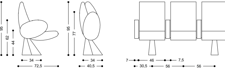
Tulip su barra - Tulip on beam
