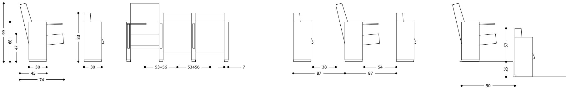
Mura “B”Vip su barra con piede centrale - Mura “B”Vip on beam with central base
