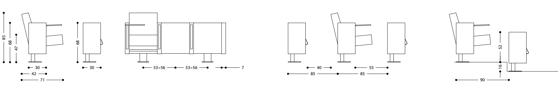
Mura “B” su barra con piede centrale - Mura “B” on beam with central base
