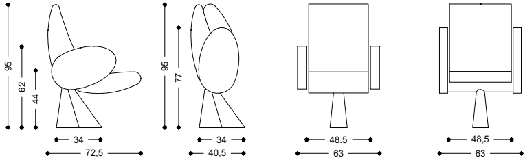
Tulip su base singola - Tulip on single base
